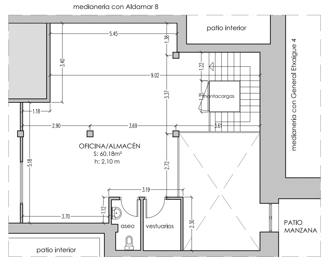
ENTREPLANTA
