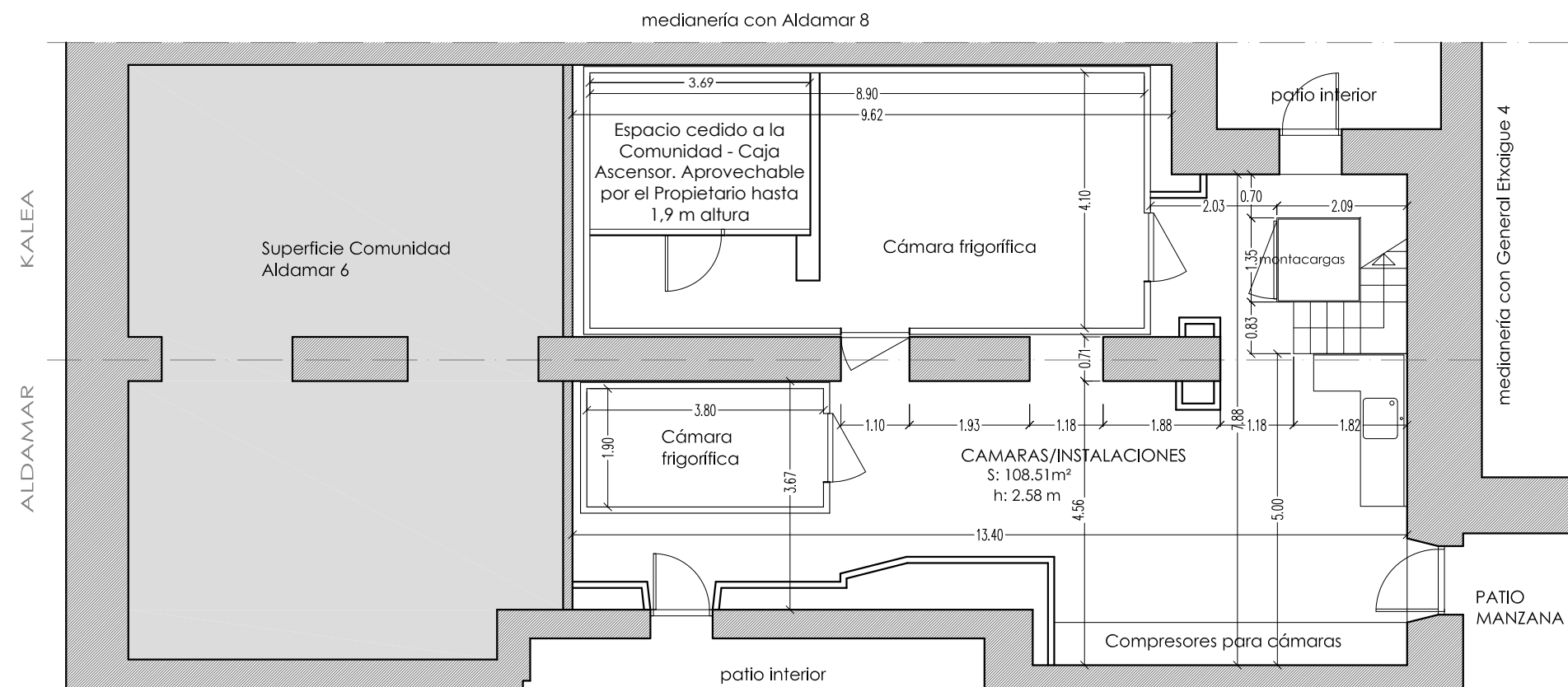
PLANTA SÓTANO
