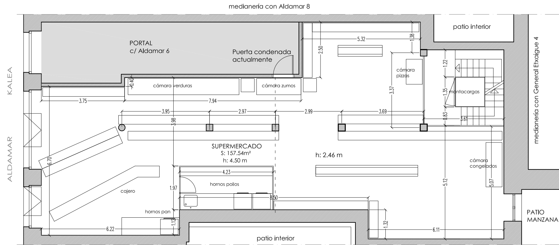
PLANTA BAJA
