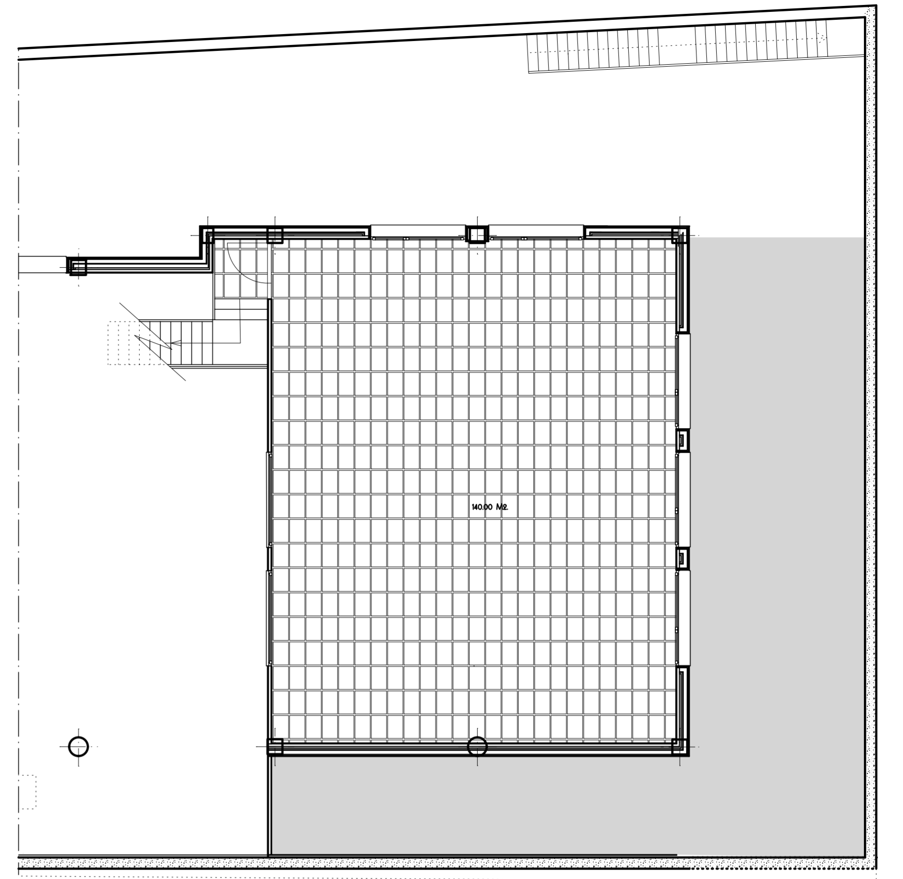
PLANTA SEMOTANO • AREA TOTAL COBERTA 800 M2
