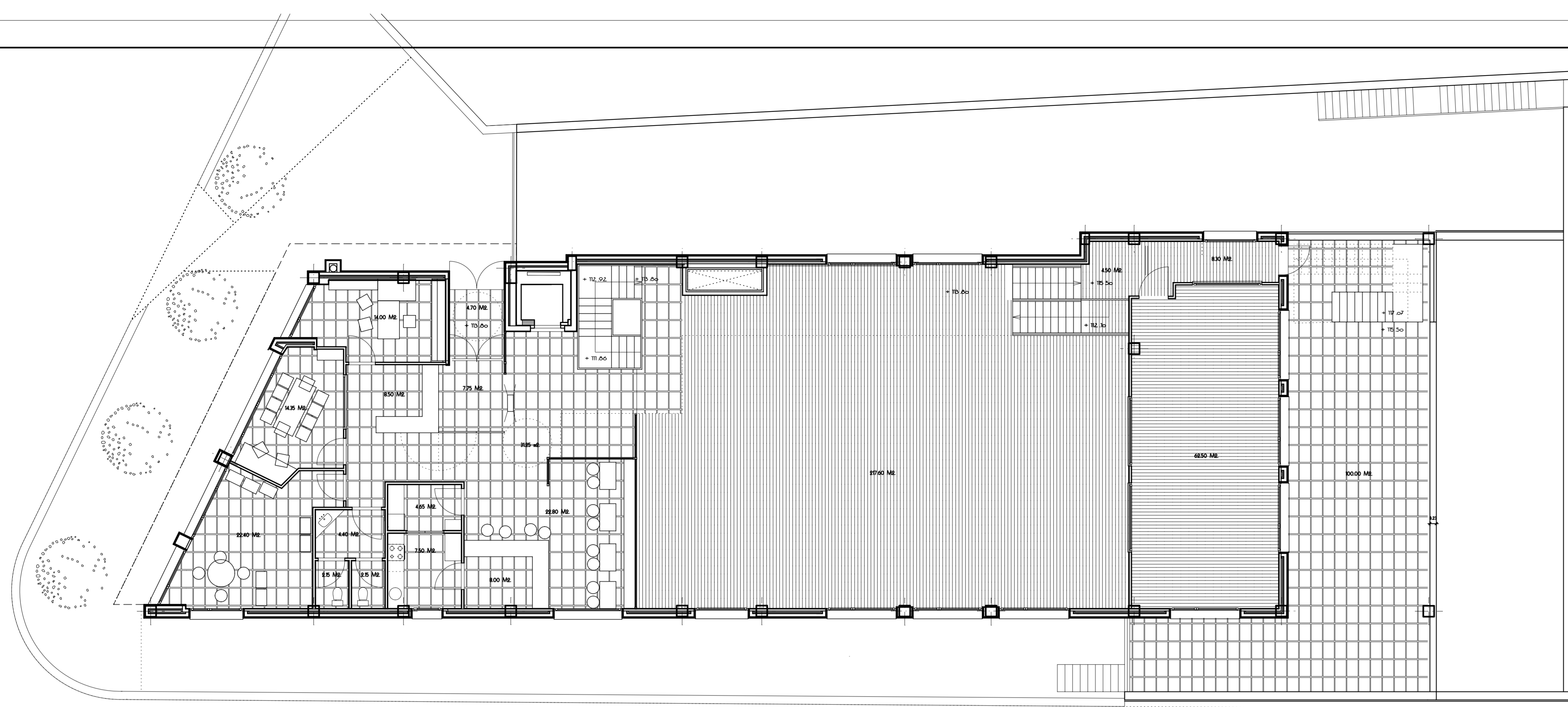
PLANTA BAJA • AREA TOTAL COBERTA 2800 M2
