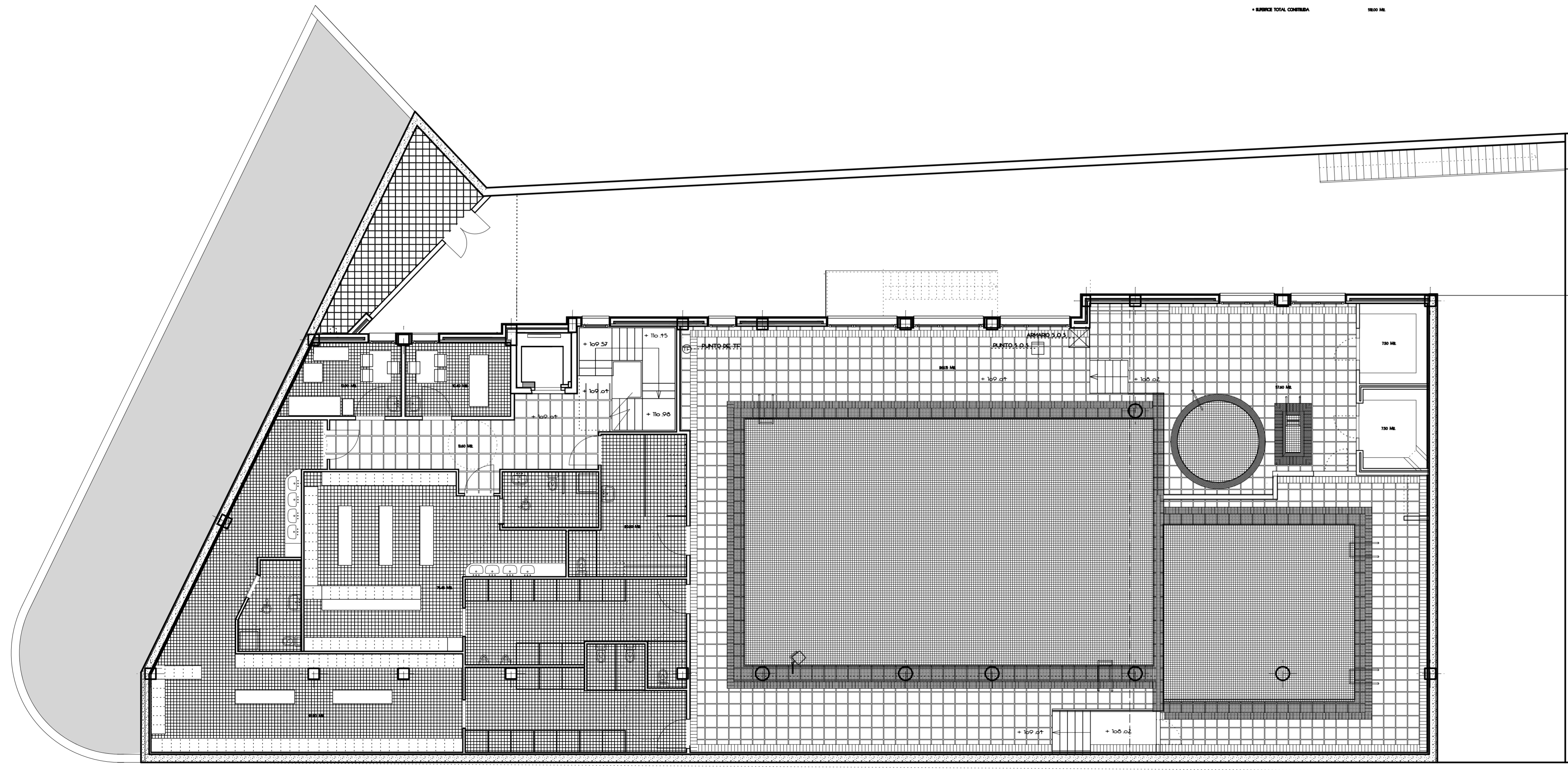
PLANTA SOTANO
