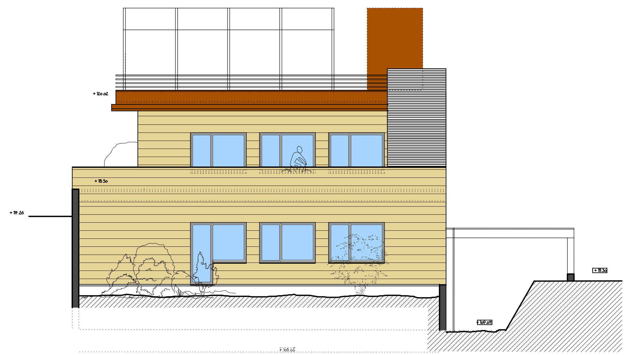
ALZADO ESTE
