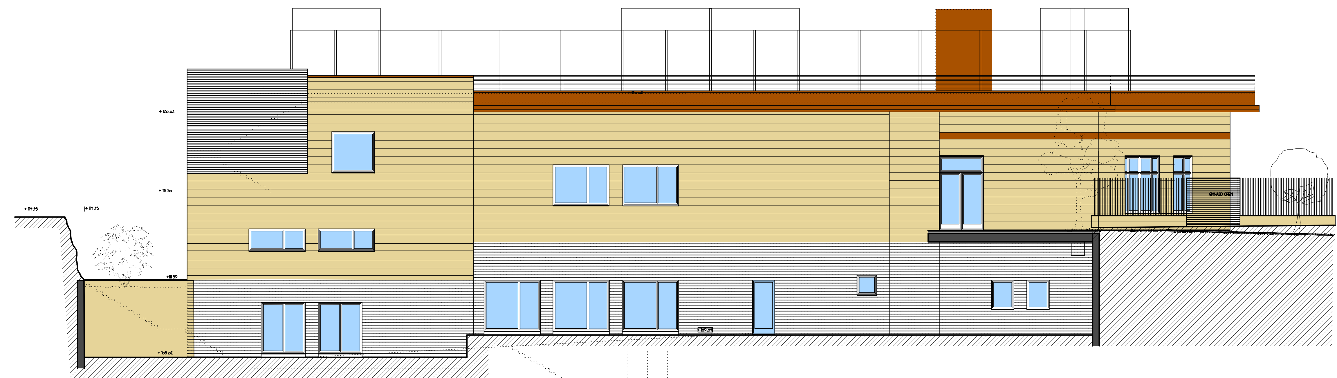
ALZADO NORTE
