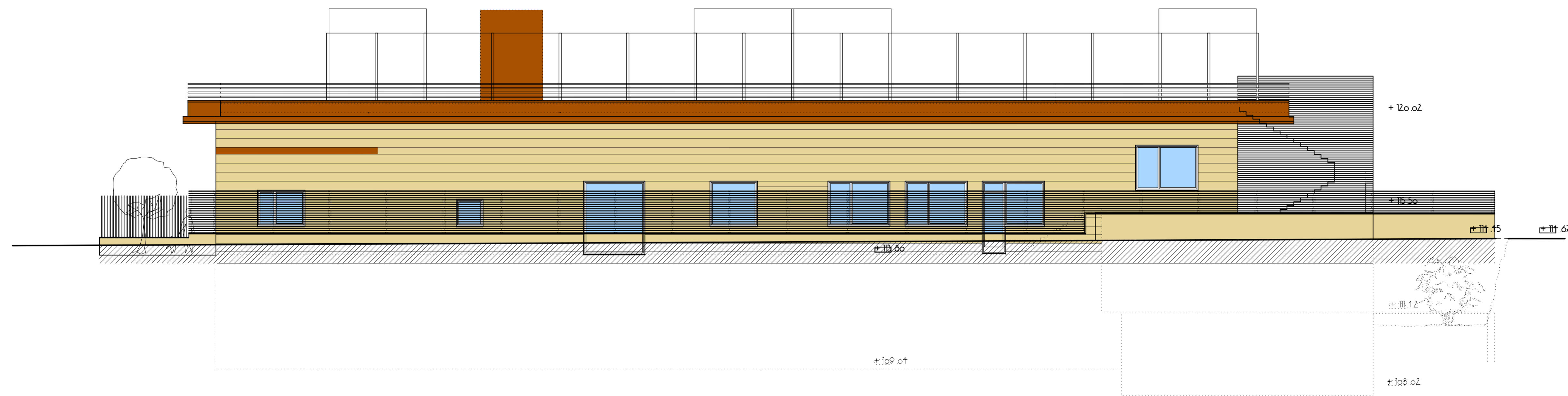
ALZADO SUR
