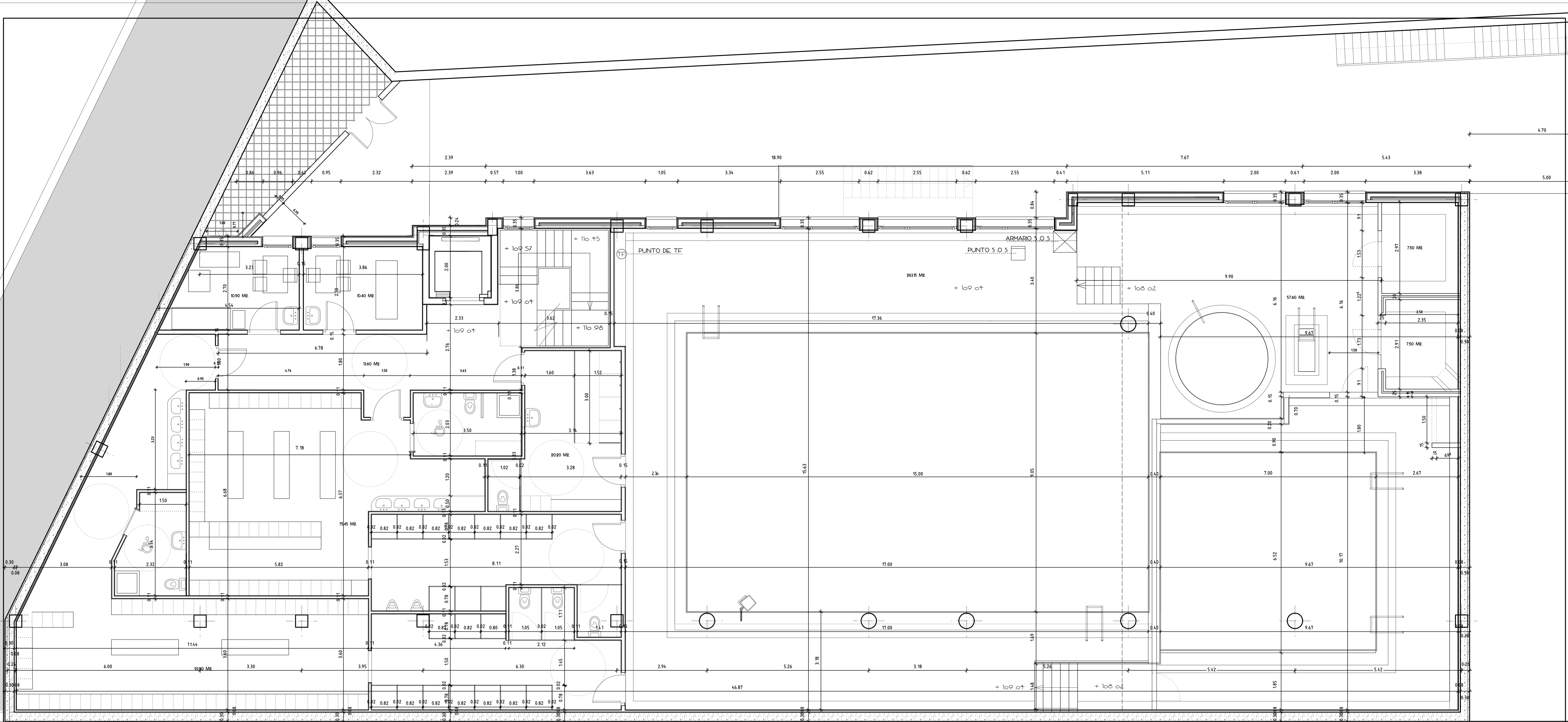
PLANTA SOTANO
